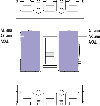
Вспомогательные контакты AXAL на EYC250
