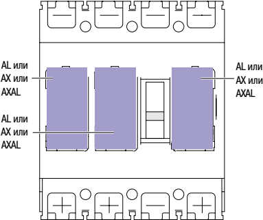
Вспомогательные контакты AXAL, AX и ALV на EYCV250
