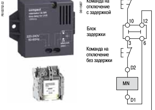
Расцепитель MN с блоком задержки
