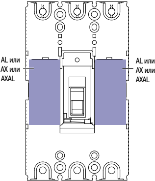
Вспомогательные контакты AXAL и AX на EYC100
